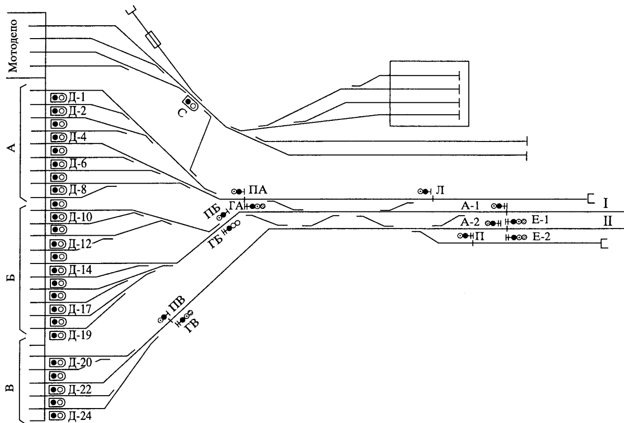
Рис. 16.2. Примерная схема парковых путей
