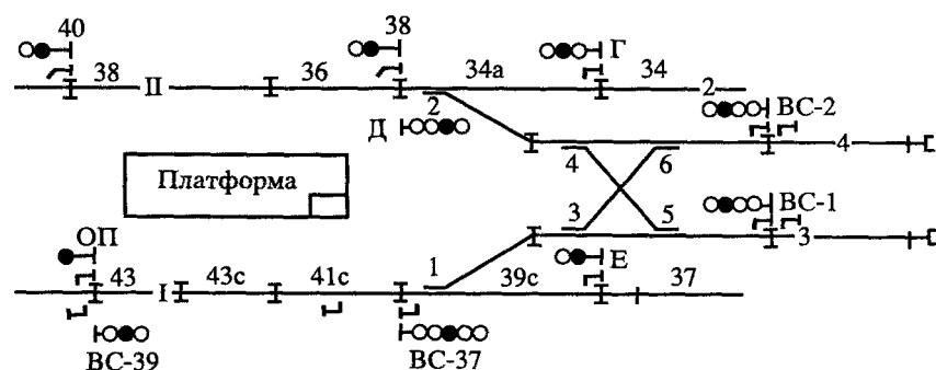
Рис. 6.6. Схема расположения предохранительных тупиковых путей
